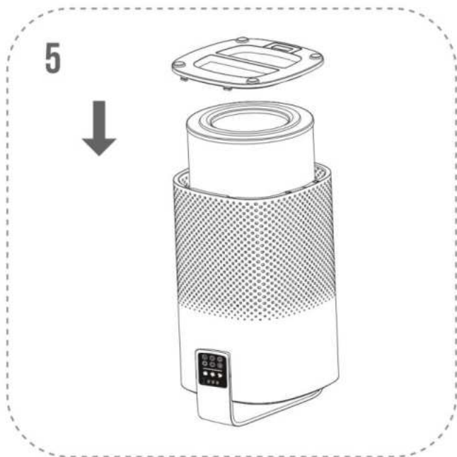
5 Włóż nowy filtr do wyłącznika. powietrze
