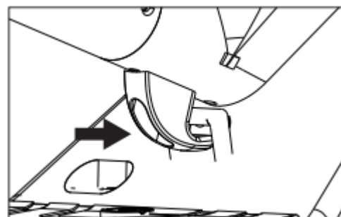
4. Împingeți ușor tija de direcție în jos pentru a cupla cârligul.
